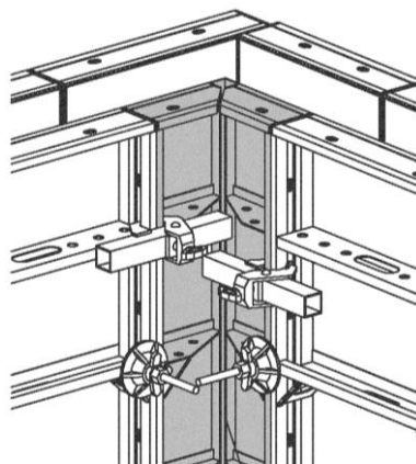
Angle Intérieur 300
