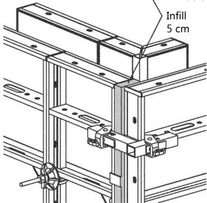
Clamp de corner
